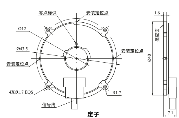
机械结构与安装图
