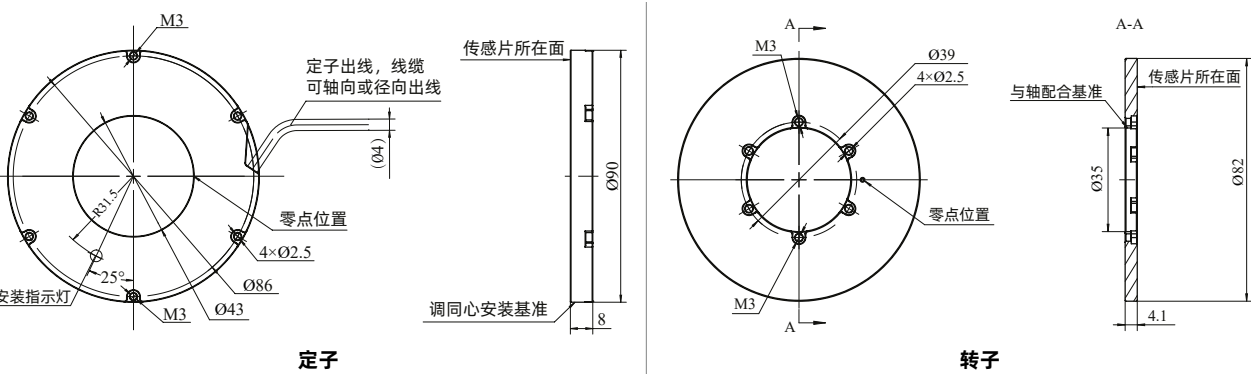
机械结构与安装图
