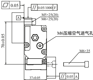
安装方向一
