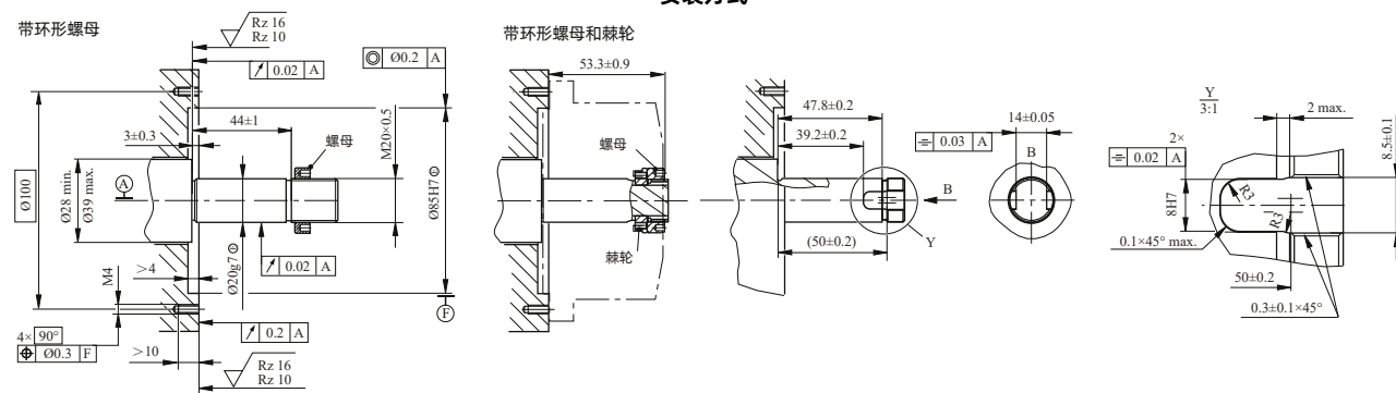
安装方式二
