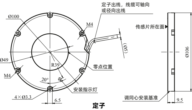
定子
