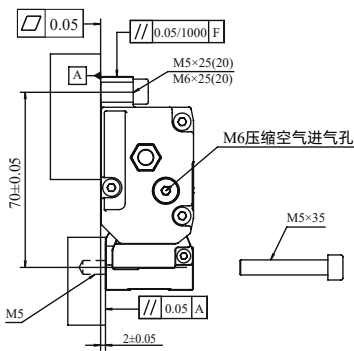
安装方向二
