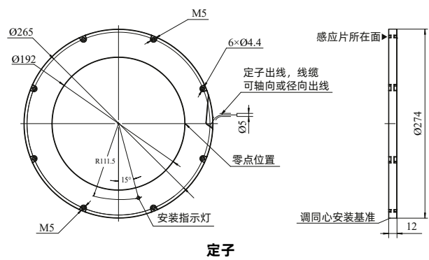
定子
