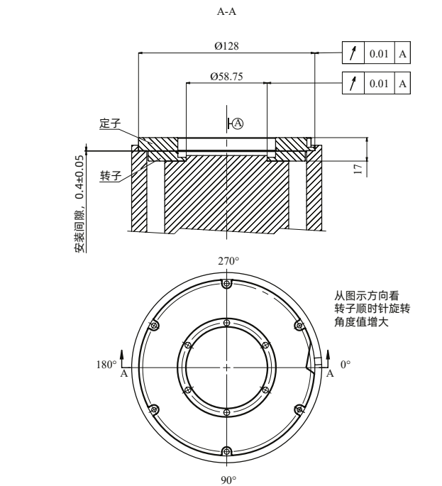
定子、转子安装相对位置
