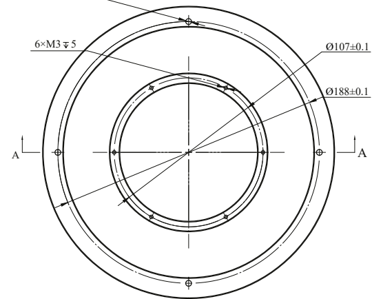
客户端安装尺寸建议
