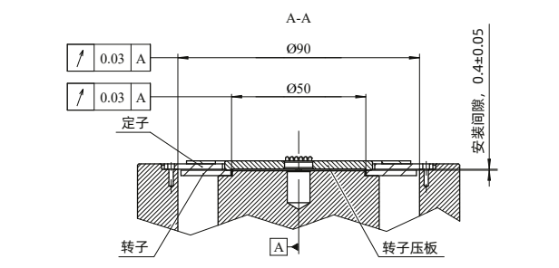
定子、转子安装相对位置
