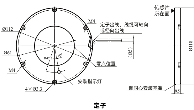
定子
