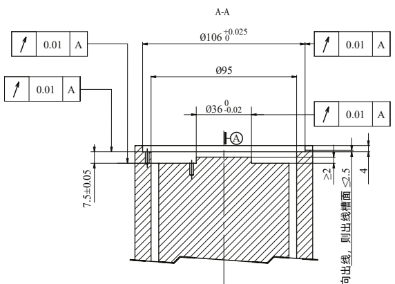
转子
