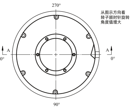
定子、转子安装相对位置
