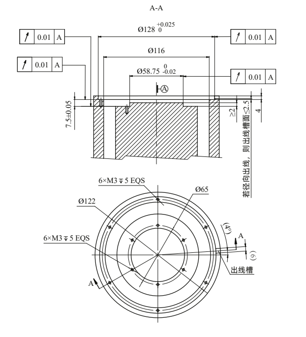
客户端安装尺寸建议
