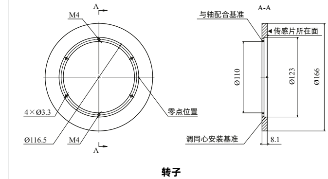
转子
