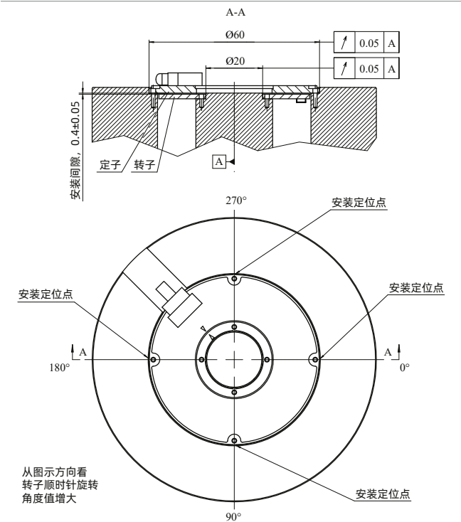
定子、转子安装相对位置
