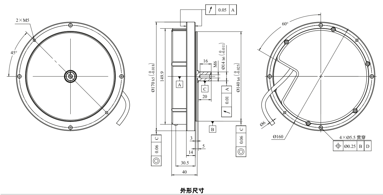
机械结构与安装图
