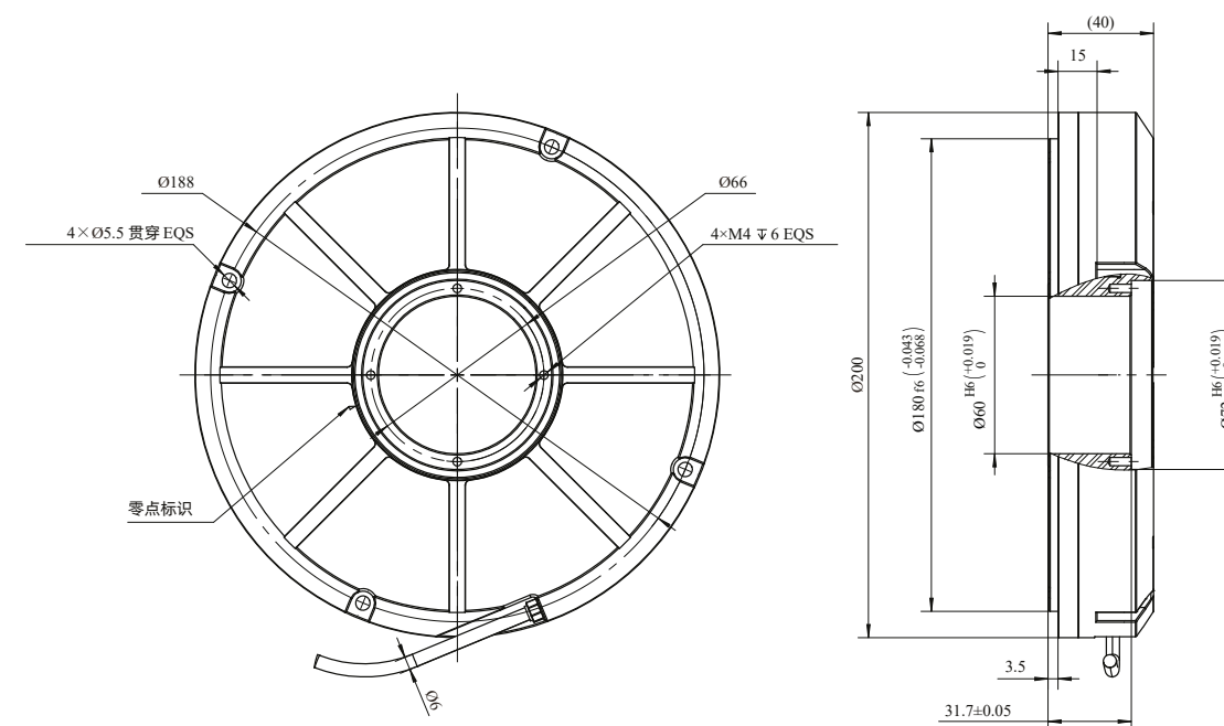
整体外形尺寸
