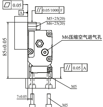
安装方向三
