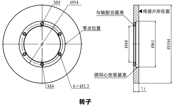
转子
