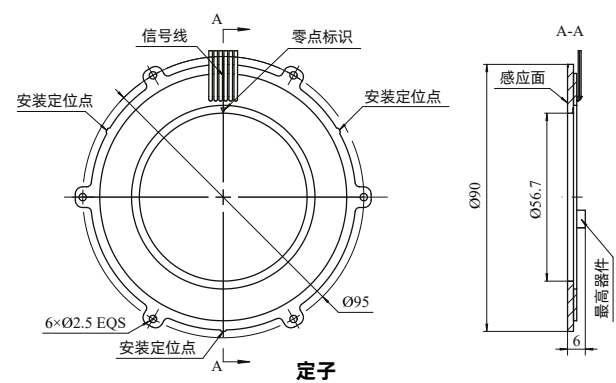
定子
