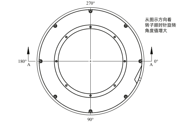
定子、转子安装相对位置
