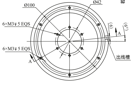
客户端安装尺寸建议
