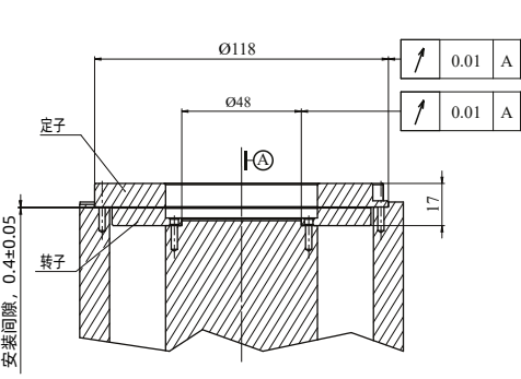
定子
