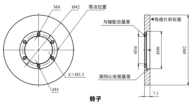
转子
