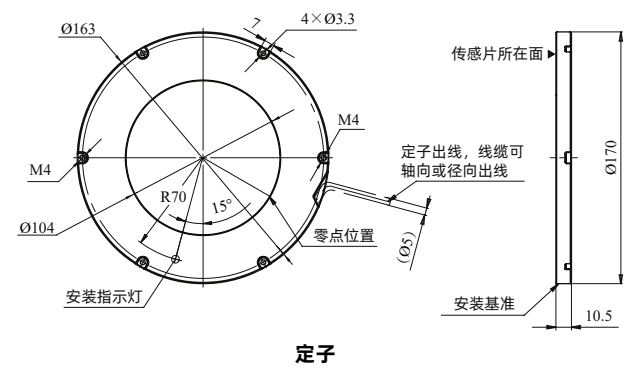
定子
