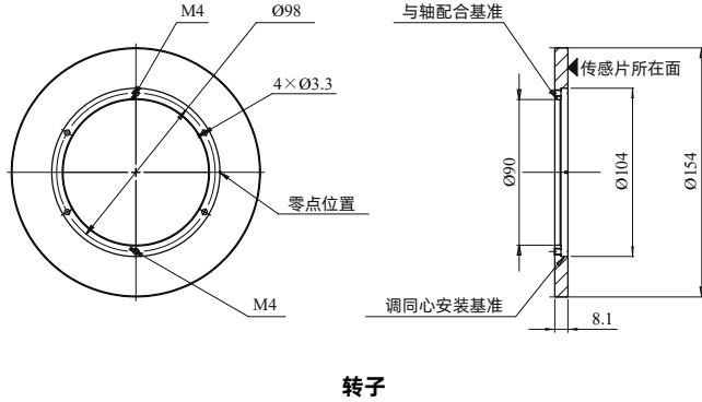
转子
