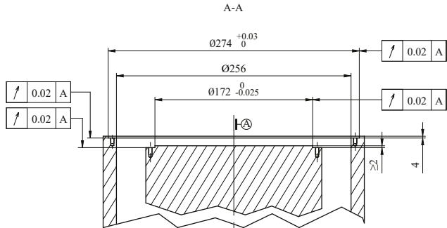
转子
