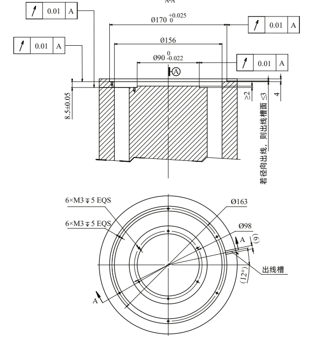
客户端安装尺寸建议
