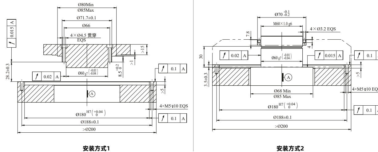
整体外形尺寸
