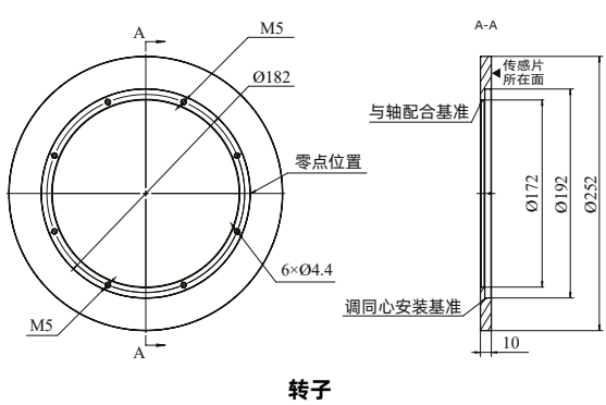
转子
