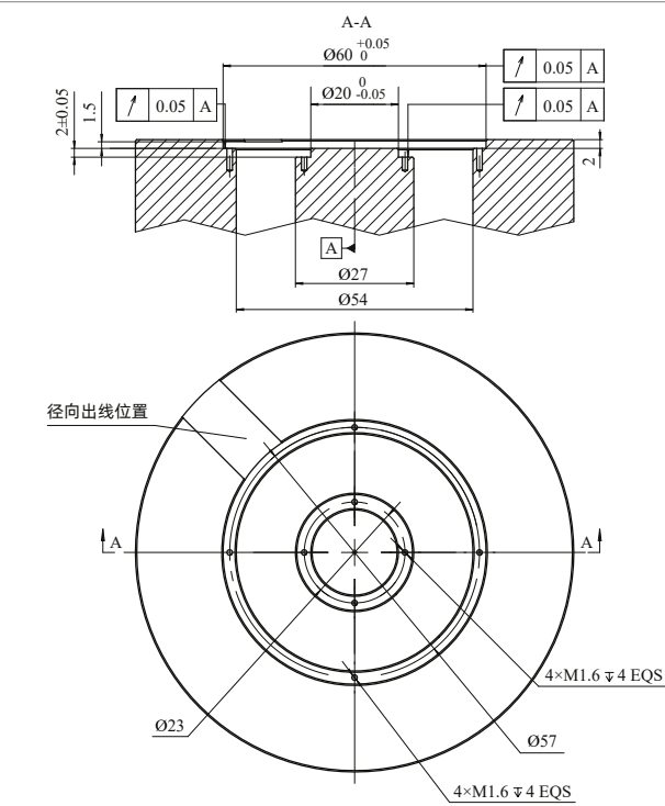
客户端安装尺寸建议
