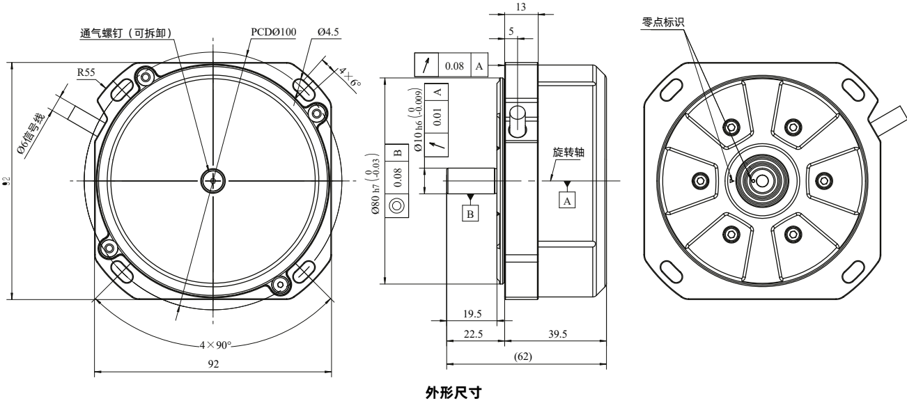
机械结构与安装图
