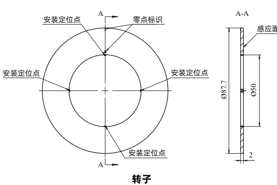
转子
